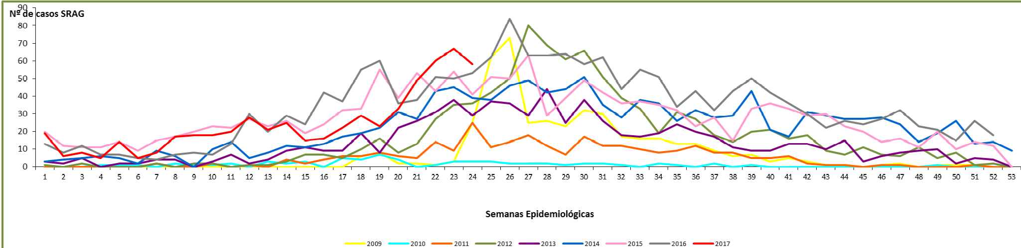
Figura 5. Número de casos de SRAG por semanas epidemiológicas de início dos sintomas, HNCS e HCC, (SE 18/2009 até SE 24/2017). Fonte NHE/HNSC-HCC. Dados sujeitos a revisão.
