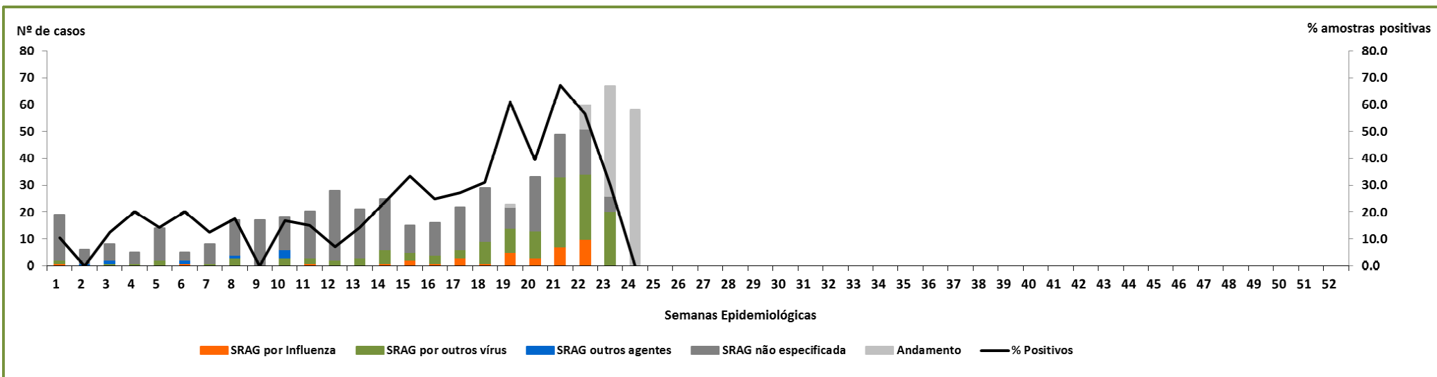
Figura 6. Número de casos de SRAG por semanas epidemiológicas de início dos sintomas, conforme a classificação final. HNCS e HCC, (SE 01/2017 a SE 24/2017). Fonte NHE/HNSC-HCC. Dados sujeitos a revisão.
