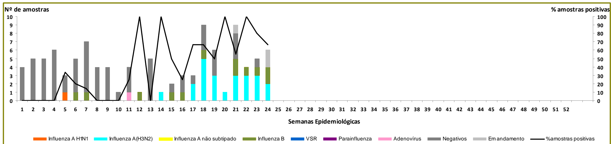
Figura 3. Tipos de vírus identificados através da Vigilância Sentinela de Síndrome Gripal por semana epidemiológica e ano de início dos sintomas, SE 01/2017 a SE 24/2017. Fonte NHE/HNSC-HCC. Dados sujeitos a revisão.
