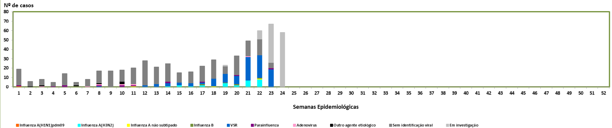
Figura 7. Número de casos de SRAG por semana epidemiológica de início dos sintomas, conforme agente etiológico. HNSC e HCC, (SE 01/2017 a SE 24/2017). Fonte NHE/HNSC-HCC. Dados sujeitos a revisão.
